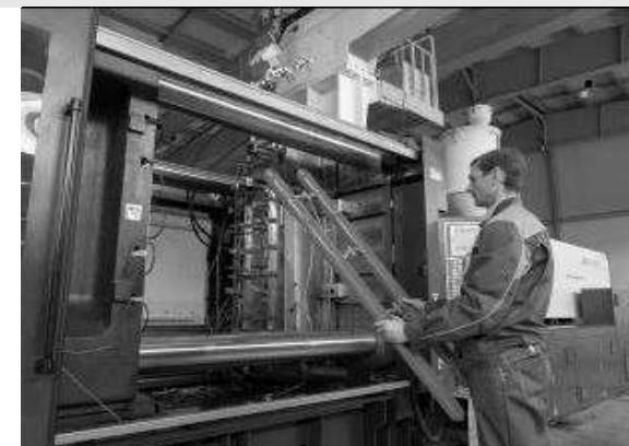
Литье пластика
